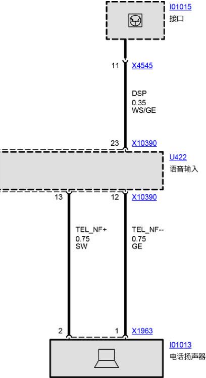
N9 收音机控制单元
